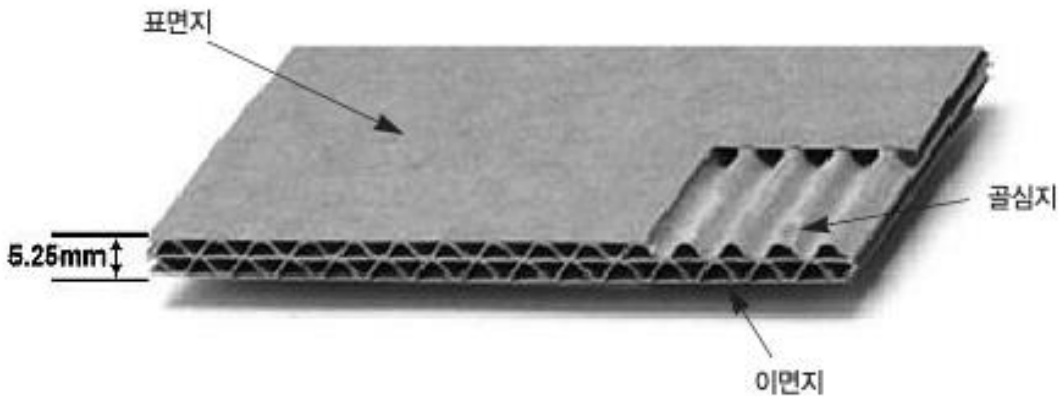
그림 1. 골판지의 구조
